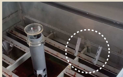
【製品テスト状況】 96時間試験後の状況(サポート)
