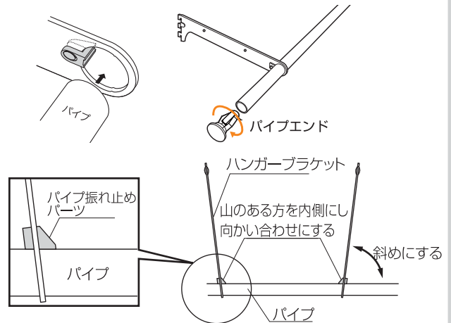
ハンガー補助パイプ (任意)
