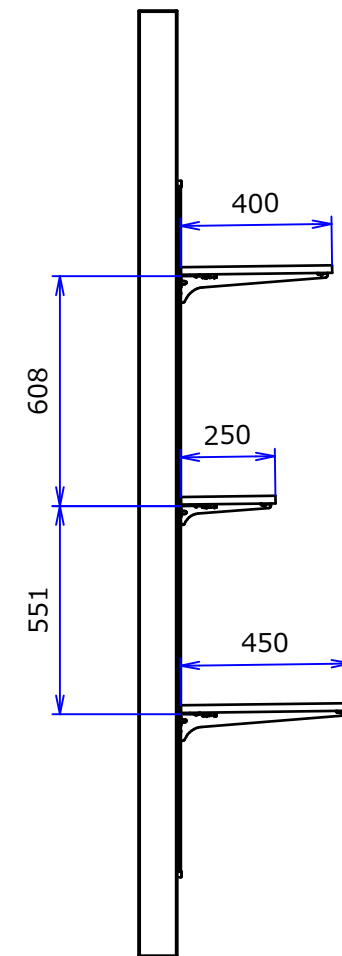
B-B ( 1 : 20 )
