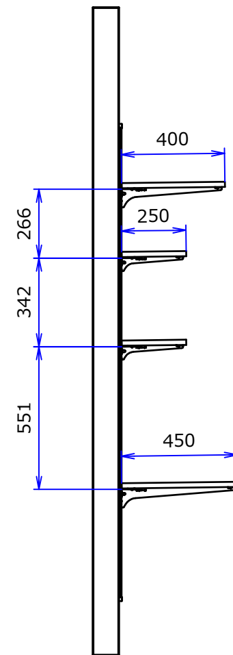
C-C ( 1 : 20 )
