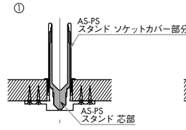
AS-PSカバー手締め作業
